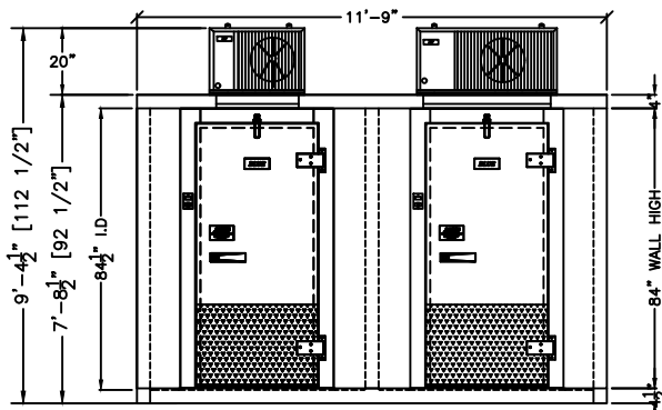
1 ELEVATION SCALE: 1/4"=1'-0"
