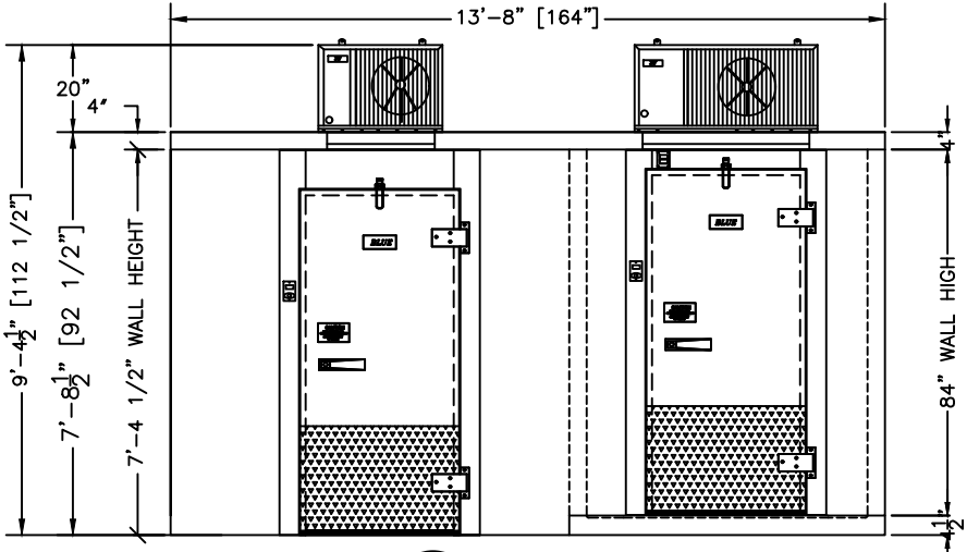
1 ELEVATION SCALE: 1/4"=1'-0"
