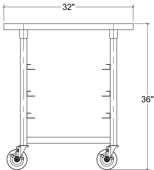
ELEVATION
