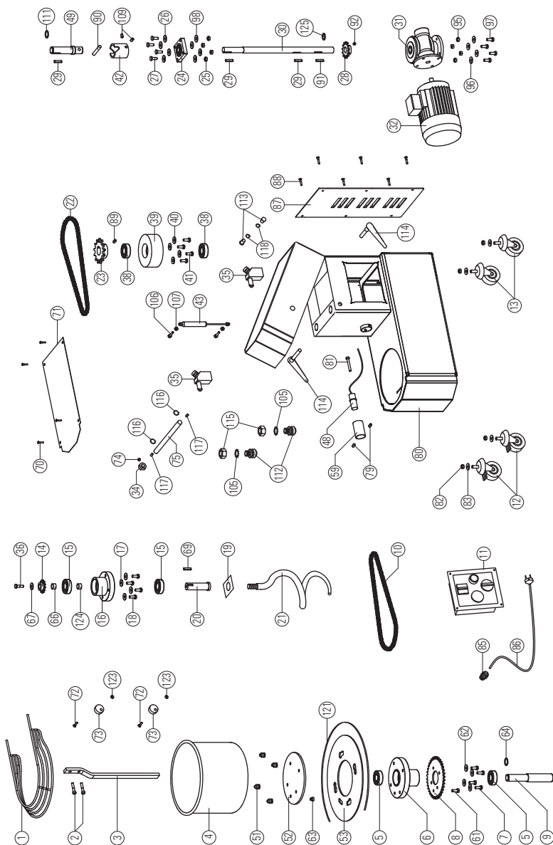
FIG. 21 Parti di ricambio impastatrice con testa sollevabile e vasca estraibile mod. IM 12-18 A FIG. 21 Pièces de rechange pour pétrisseuse avec tête soulevable et cuve extractible mod. IM 12-18 A PICT. 21 Spare parts for mixer with raising top and removable bowl mod. IM 12-18 A BILD 21 Ersatzteile für die Teigknetmaschine mit hebbaarem Kopf und herausziehbarem Becken mod. IM 12-18 A
