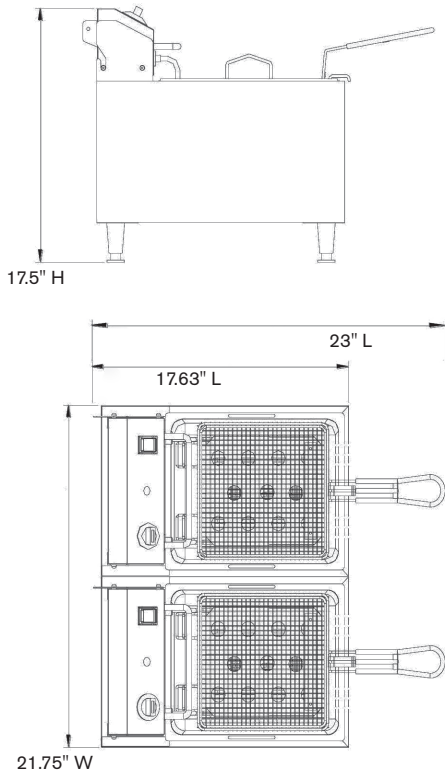
PF32E-C
