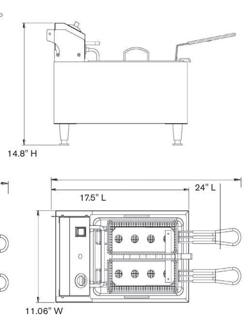
PF10E-C
