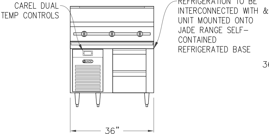
ELEVATION
