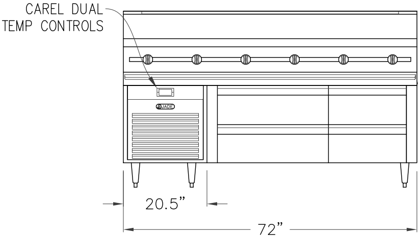
ELEVATION
