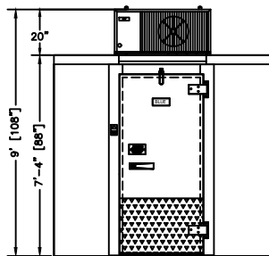
ELEVATION RIGHT HINGE
