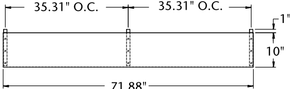
PLAN VIEW NLSP72-18A, NLSMP72-30A
