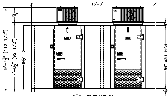
1 ELEVATION SCALE: 1/4"=1'-0"
