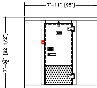
ELEVATION RIGHT HINGE
