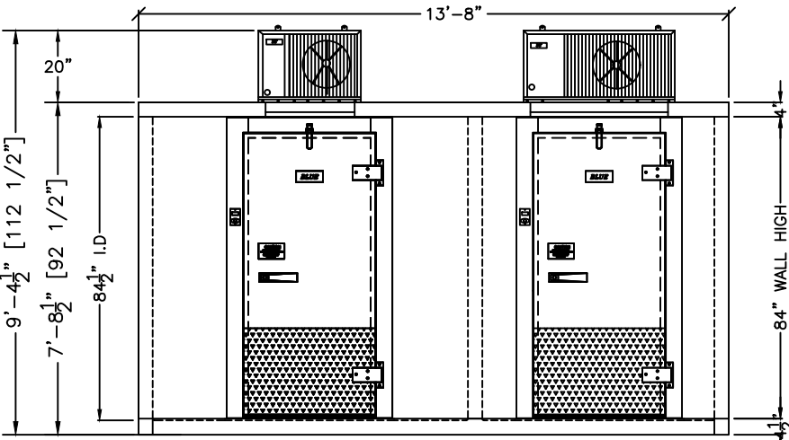
1 ELEVATION SCALE: 1/4"=1'-0"
