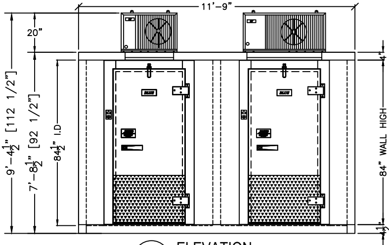
1 ELEVATION SCALE: 1/4"=1'-0"
