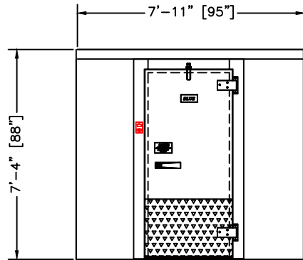
ELEVATION RIGHT HINGE
