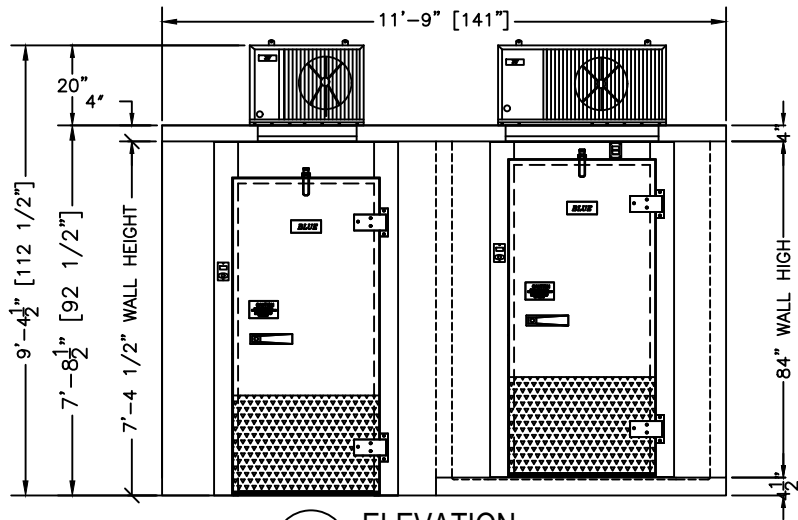
1 ELEVATION SCALE: 1/4"=1'-0"
