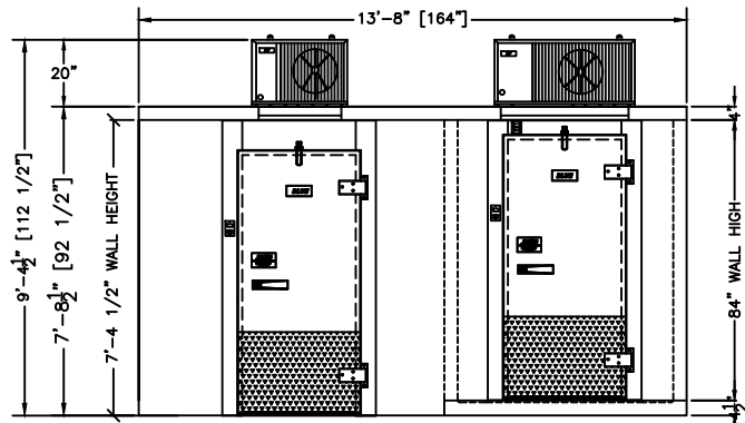
1 ELEVATION SCALE: 1/4"=1'-0"
