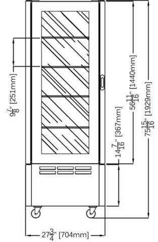
VC6314D H76 & VC8314D H76
