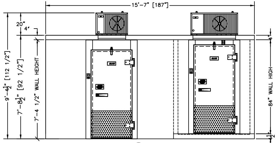
1 ELEVATION SCALE: 1/4"=1'-0"
